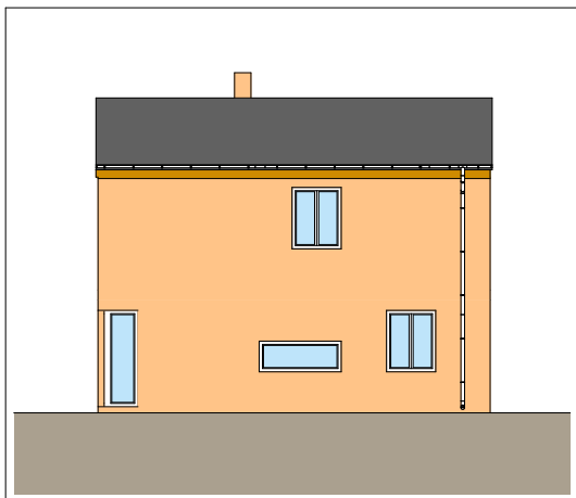
Zahradní pohled:
